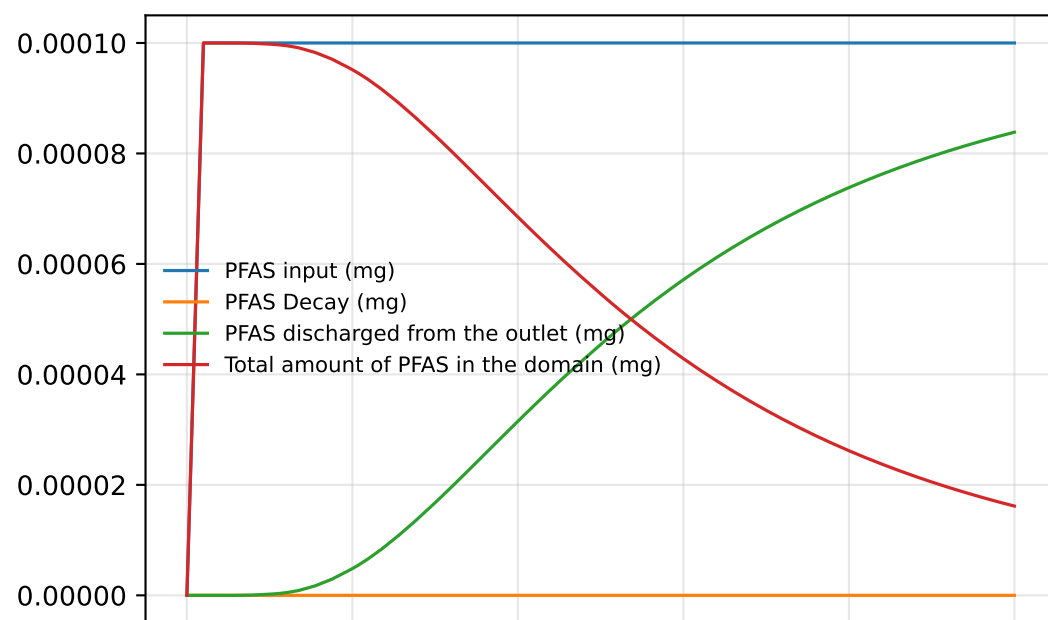
PFAS Balance
